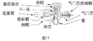
图11 将截止阀打开，使制冷剂可从室外机组流至室内机组
