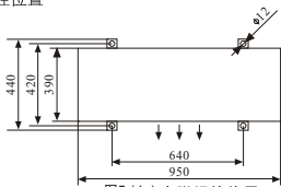
图5 (b) 底脚螺栓位置
